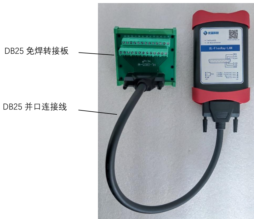
图 5 DB25 免焊转接板使用说明实物图
